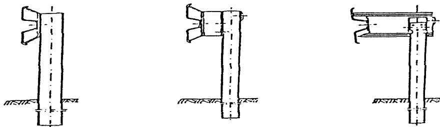
Załącznik 11.2 Bariery ochronne stalowe skrajne z prowadnicą z profilowanej taśmy stalowej stosowane na odcinkach dróg, według [32]
